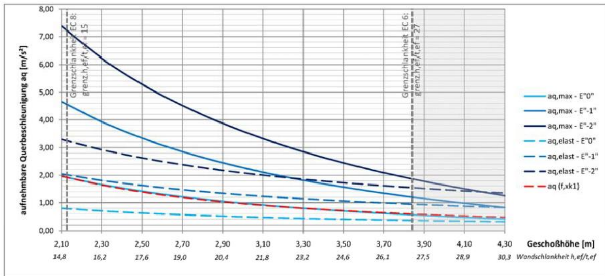
Bild 5: mögliche Querbeschleunigungen von Aussteifungswänden
